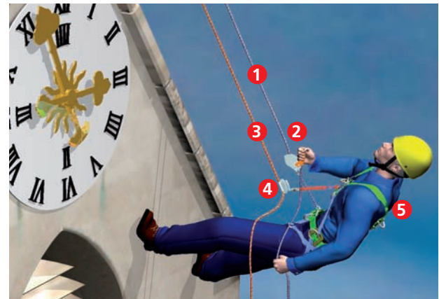
Zugangs- und Arbeitsplatzpositionierungssystem auf geneigter oder senkrechter Fläche
