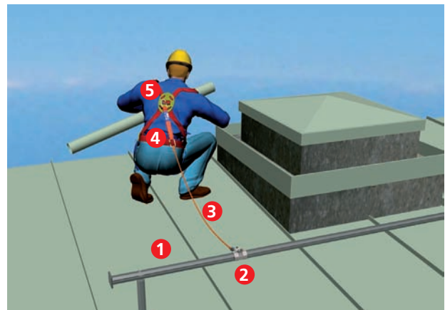
Auffangsystem mit Falldämpfer und horizontaler Anschlagseinrichtung
