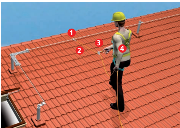
Auffangsystem mit mitlaufendem Auffanggerät einschließlich beweglicher Führung und horizontaler Anschlagseinrichtung
